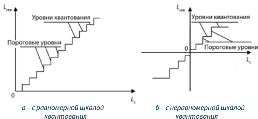
Рисунок 6 – Амплитудные характеристики квантующих устройств
